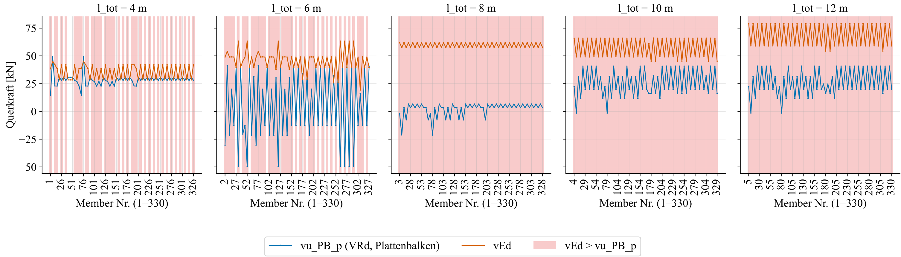
Querkraftwiderstand v_{u\_PB\_p} (VRd, Plattenbalken) vs. Bemessungsquerkraft v_{Ed} je Member, kategorisiert nach Spannweite (Members_rc_rib_simple_)
